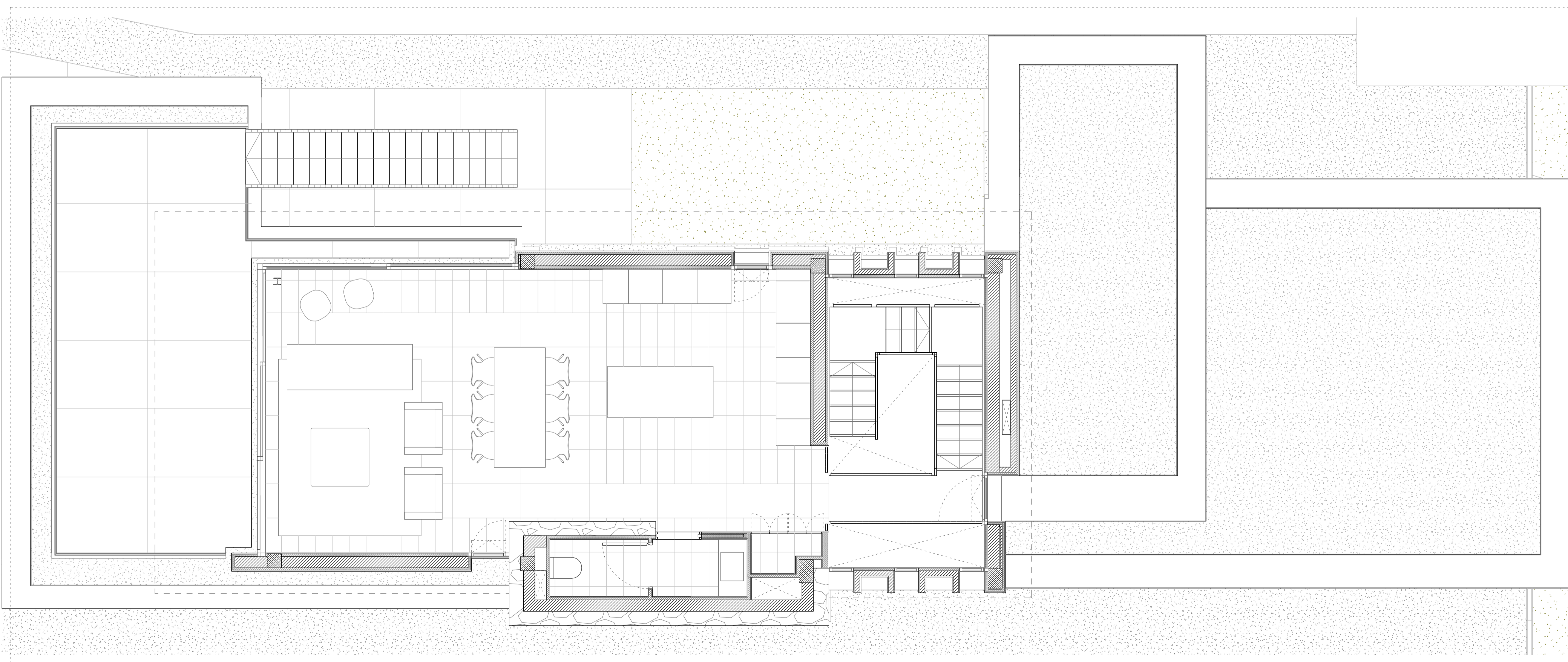
PLANTA PRIMERA
